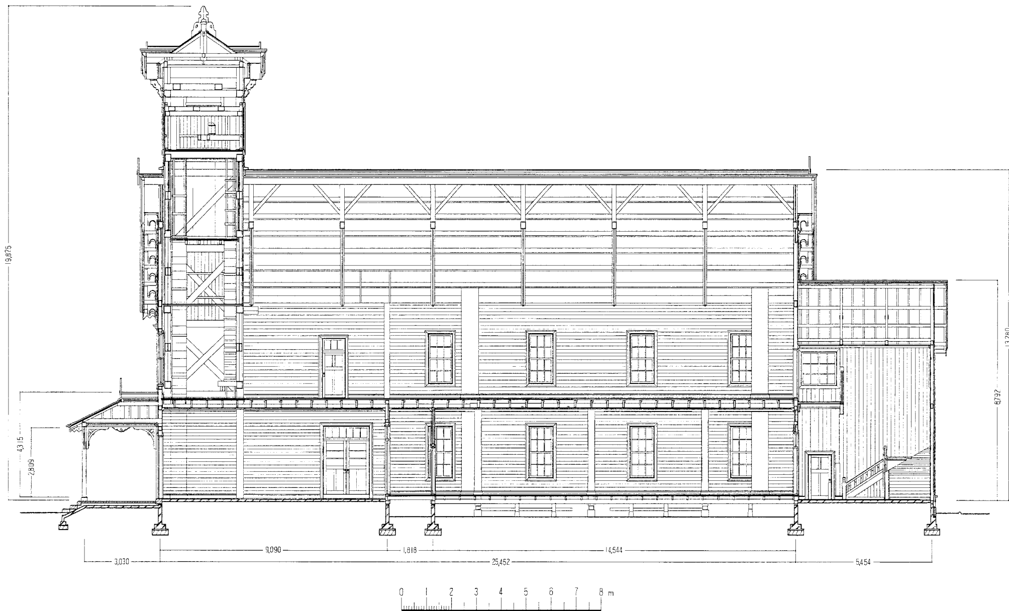
7. 竣工 桁行断面图
