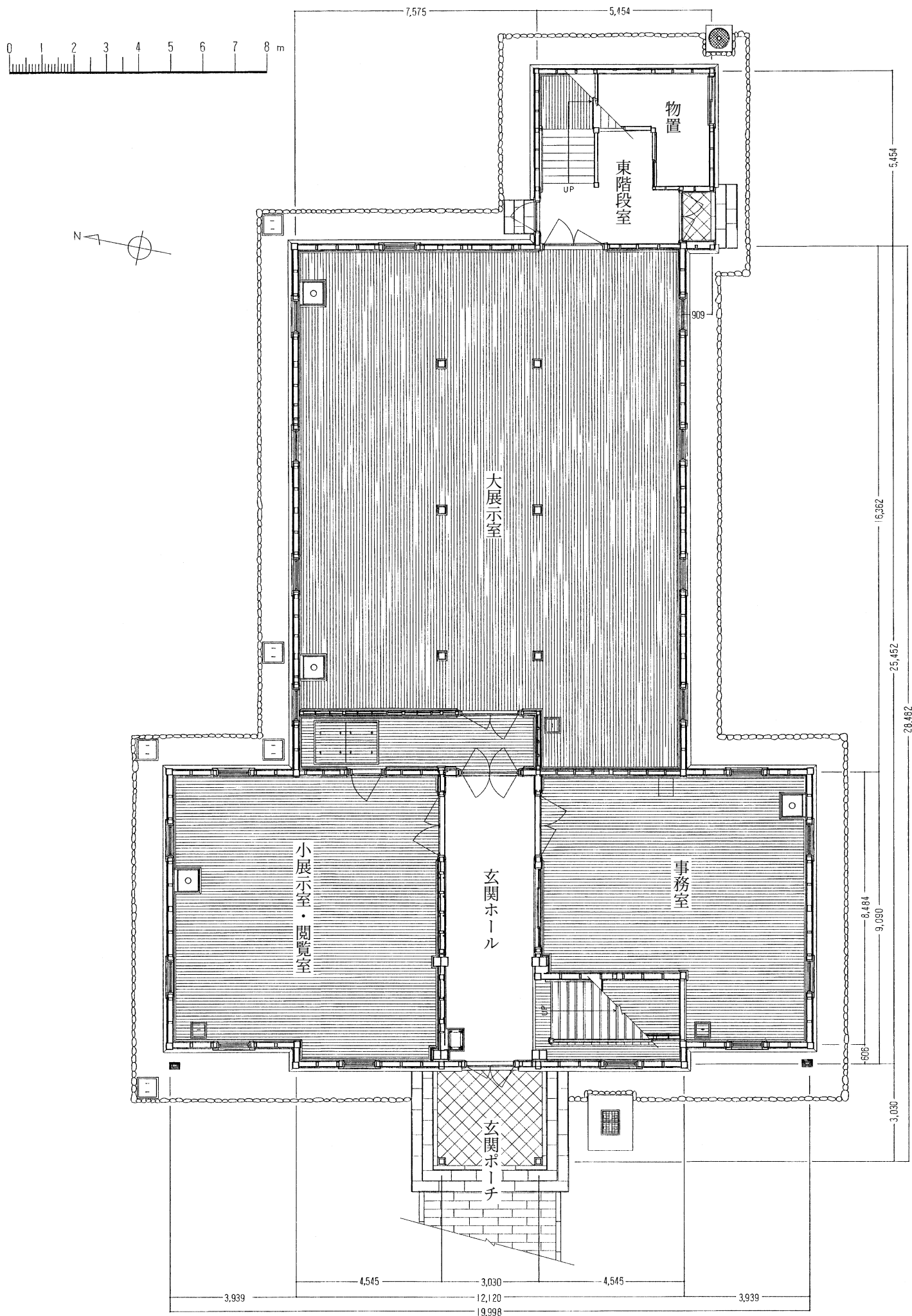
1. 竣工 1階平面図
