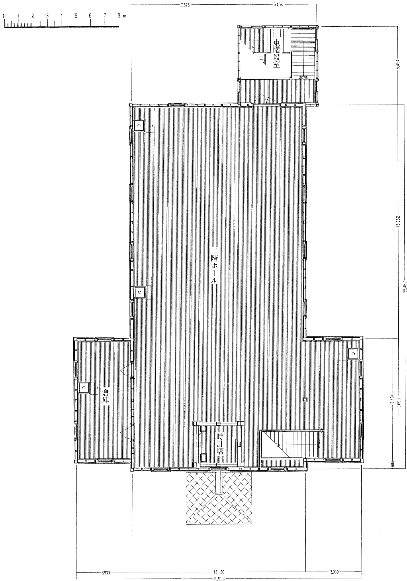
2. 竣工 2階平面図
